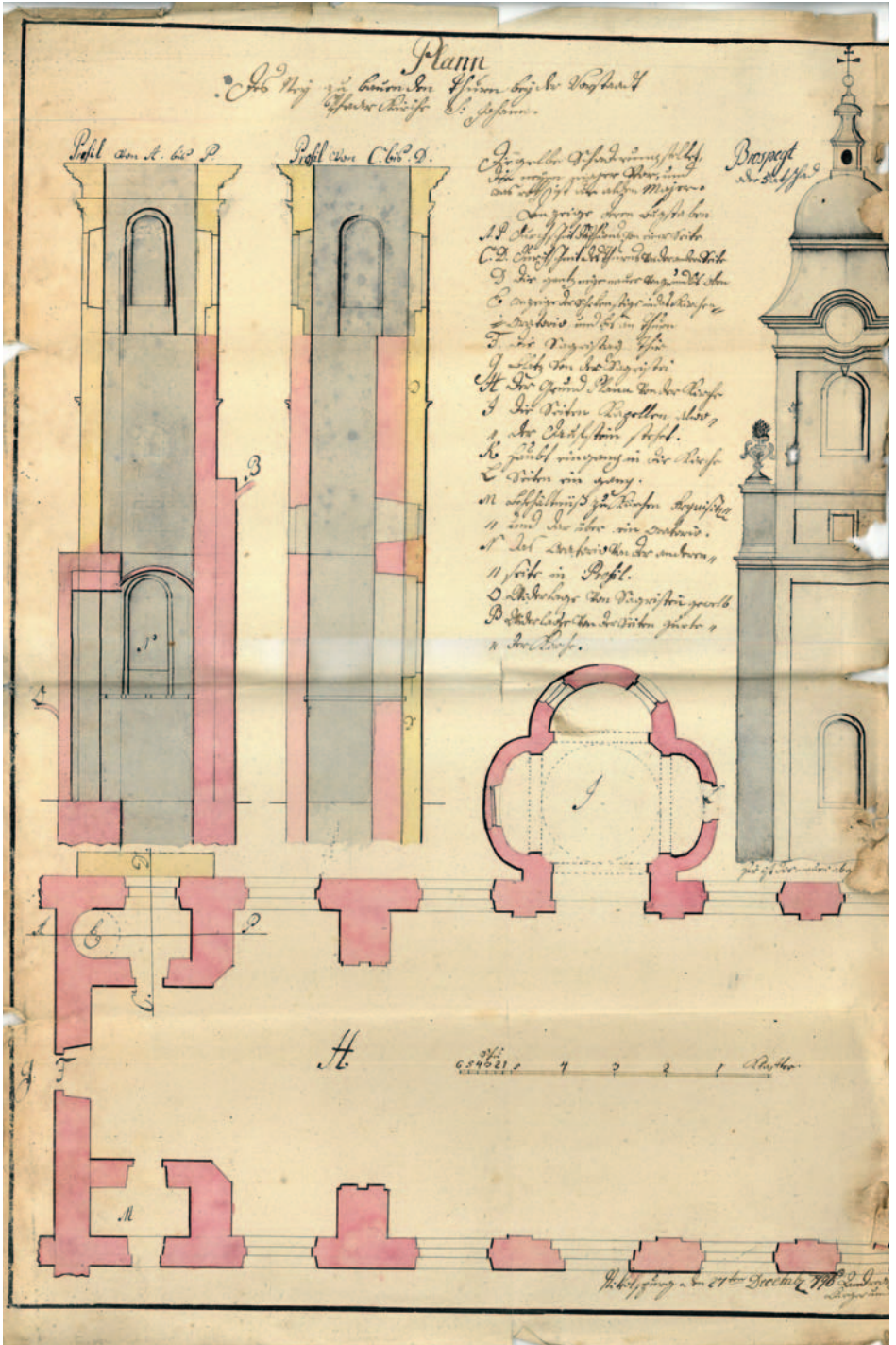
Plán věže - Ondřej Rieder 1796 (Diecézní archiv Biskupství brněnského, fond Farní úřad při kostele sv. Jana Mikulov)
