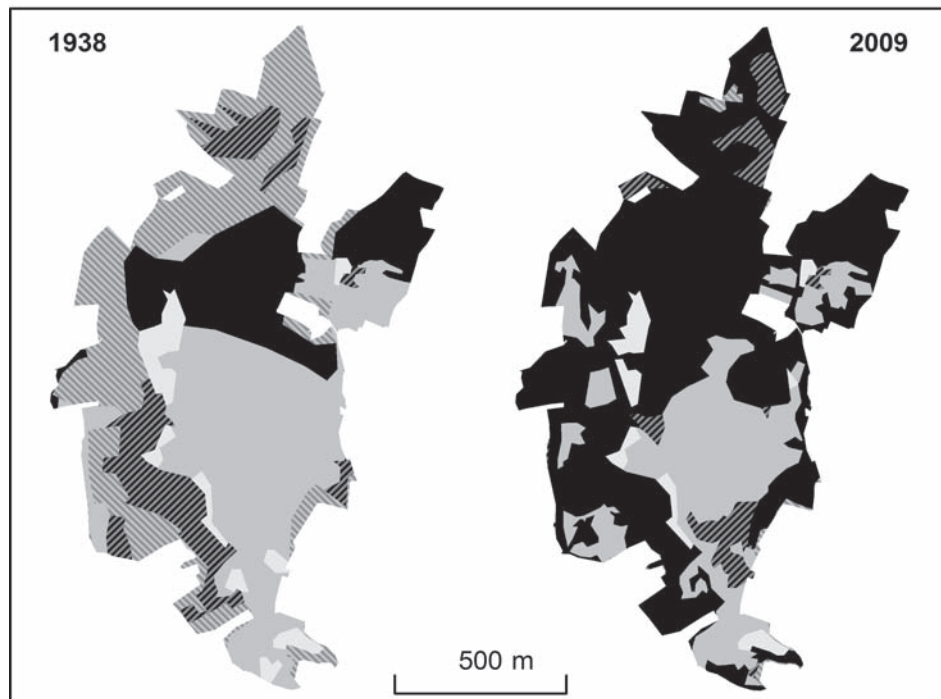
Využití území/krajinný pokryv v NPR Děvín-Kotel-Soutěska (nahoře) a NPR Tabulová v letech 1938 a 2009
