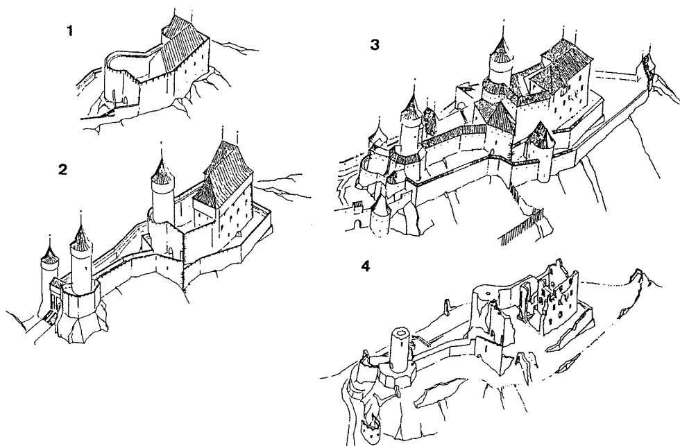
Obr. 2 - Hrad Nový Cimburk - nákresy perspektivních pohledů od jihovýchodu: 1 - rekonstrukce hradního jádra před polovinou 14. století; 2 - rekonstrukce hradu na konci 14. století; 3 - rekonstrukce hradu v 16. století (mimo kresbu vlevo je předsunutá bašta); 4 - dnešní stav areálu
